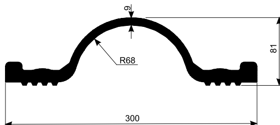
Taśma uszczelniająca do przerw dylatacyjnych zewnętrzna NX
