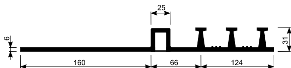
Taśma uszczelniająca do przerw dylatacyjnych zewnętrzna EX
