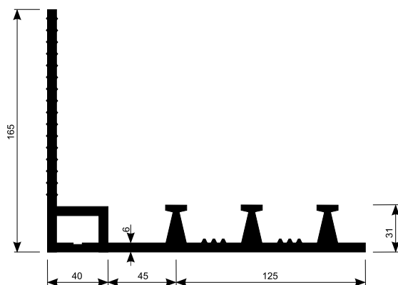
Taśma uszczelniająca do przerw dylatacyjnych zewnętrzna EX
