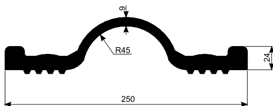
Taśma uszczelniająca do przerw dylatacyjnych zewnętrzna NX
