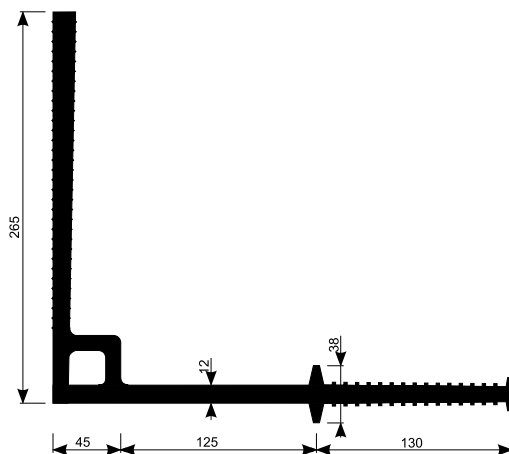
Taśma uszczelniająca do przerw dylatacyjnych wewnętrzna EX
