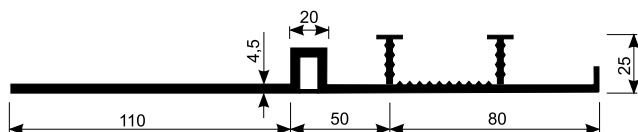
Taśma uszczelniająca do przerw dylatacyjnych zewnętrzna NX
