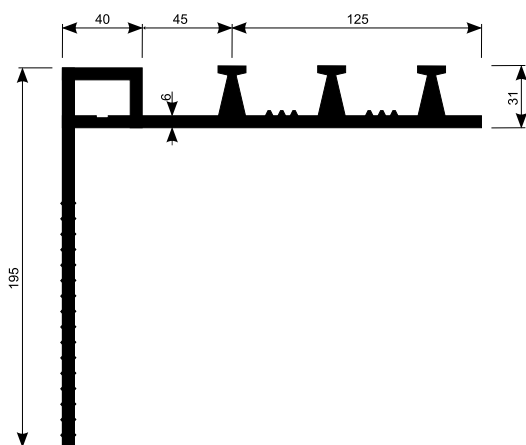
Taśma uszczelniająca do przerw dylatacyjnych zewnętrzna EX
