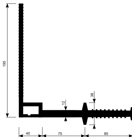
Taśma uszczelniająca do przerw dylatacyjnych wewnętrzna EX
