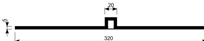
Taśma uszczelniająca do przerw dylatacyjnych zewnętrzna NX
