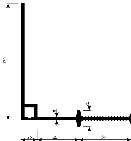
Taśma uszczelniająca do przerw dylatacyjnych wewnętrzna NX
