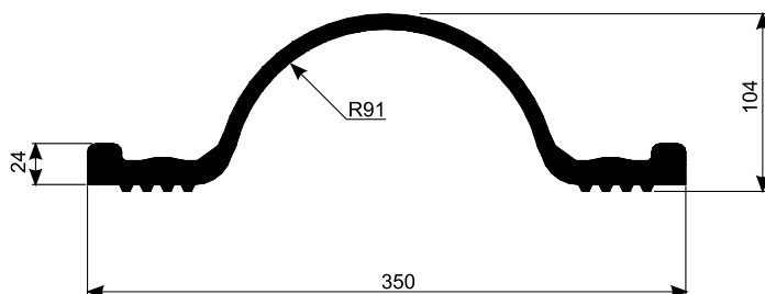
Taśma uszczelniająca do przerw dylatacyjnych zewnętrzna NX
