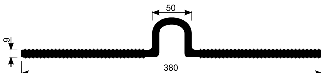
Taśma uszczelniająca do przerw dylatacyjnych zewnętrzna EX
