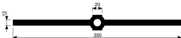
Taśma uszczelniająca do przerw dylatacyjnych zewnętrzna EX
