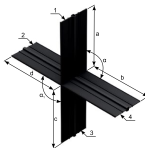
Kształtka połączeniowa przestrzenna typ X
