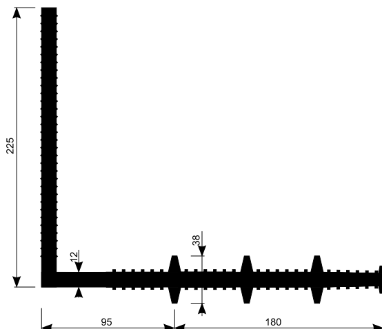
Taśma uszczelniająca do przerw dylatacyjnych wewnętrzna EX
