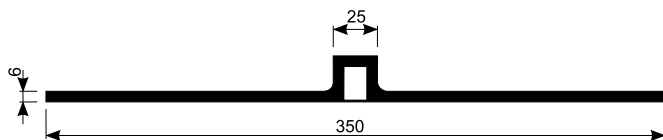
Taśma uszczelniająca do przerw dylatacyjnych zewnętrzna EX
