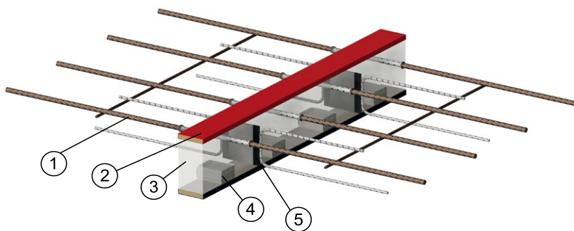
Ogólna budowa łączników FBZ
