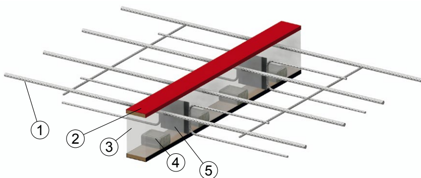
Ogólna budowa łączników FB
