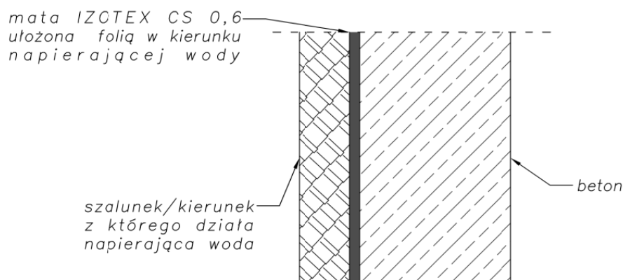
Schemat montażu maty IZOTEX CS 0,6
